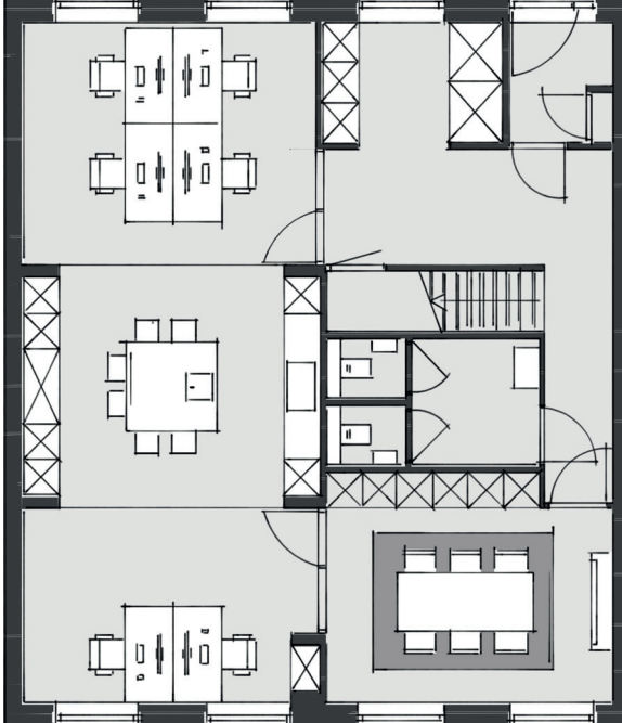
BEGANE GROND
